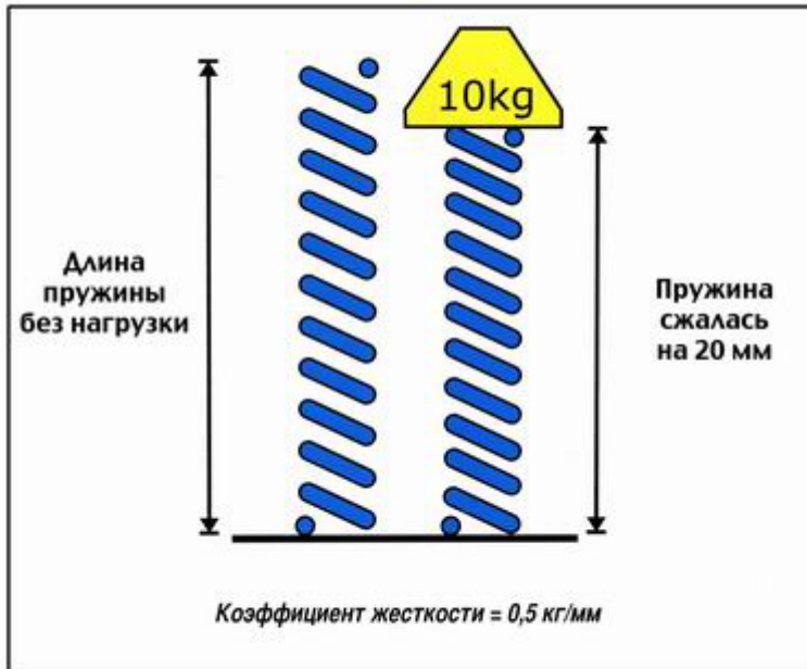
РИСУНОК 2: КОЭФФИЦИЕНТ ЖЕСТКОСТИ
